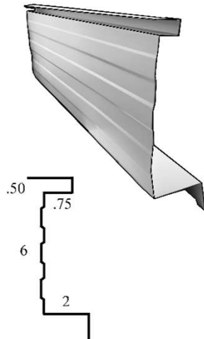
6" Divider Frieze
